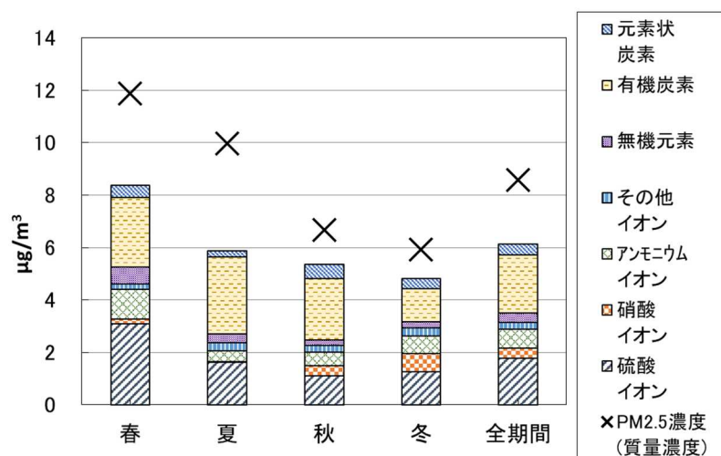
各季節の PM2.5 成分構成
