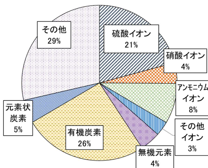
PM2.5 成分構成比（全期間平均）
