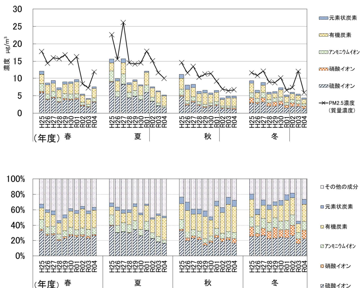
各季節における PM2.5 成分の濃度推移および成分割合推移
